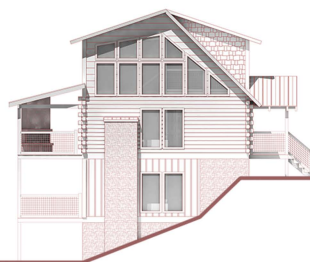
Right Elevation
