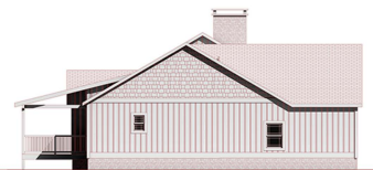
Right Elevation
