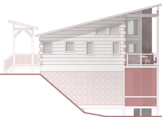
Right Elevation
